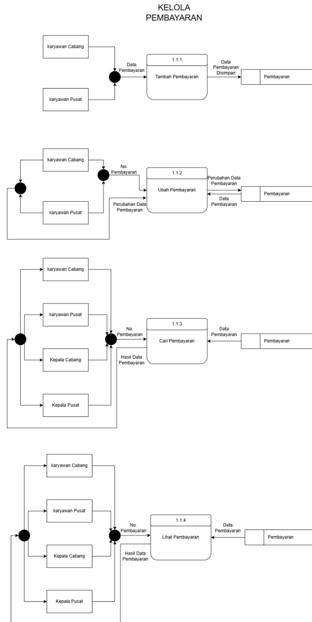
Gambar 4.32 Data Flow Diagram Pembayaran
