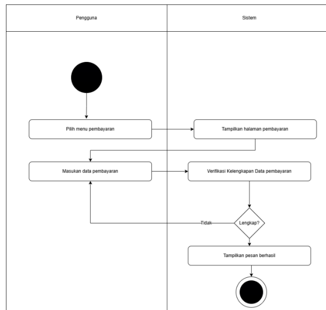
Gambar 1.10 Activity Diagram Tambah Pembayaran
