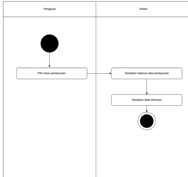
Gambar 1.13 Activity Diagram Lihat Pembayaran
