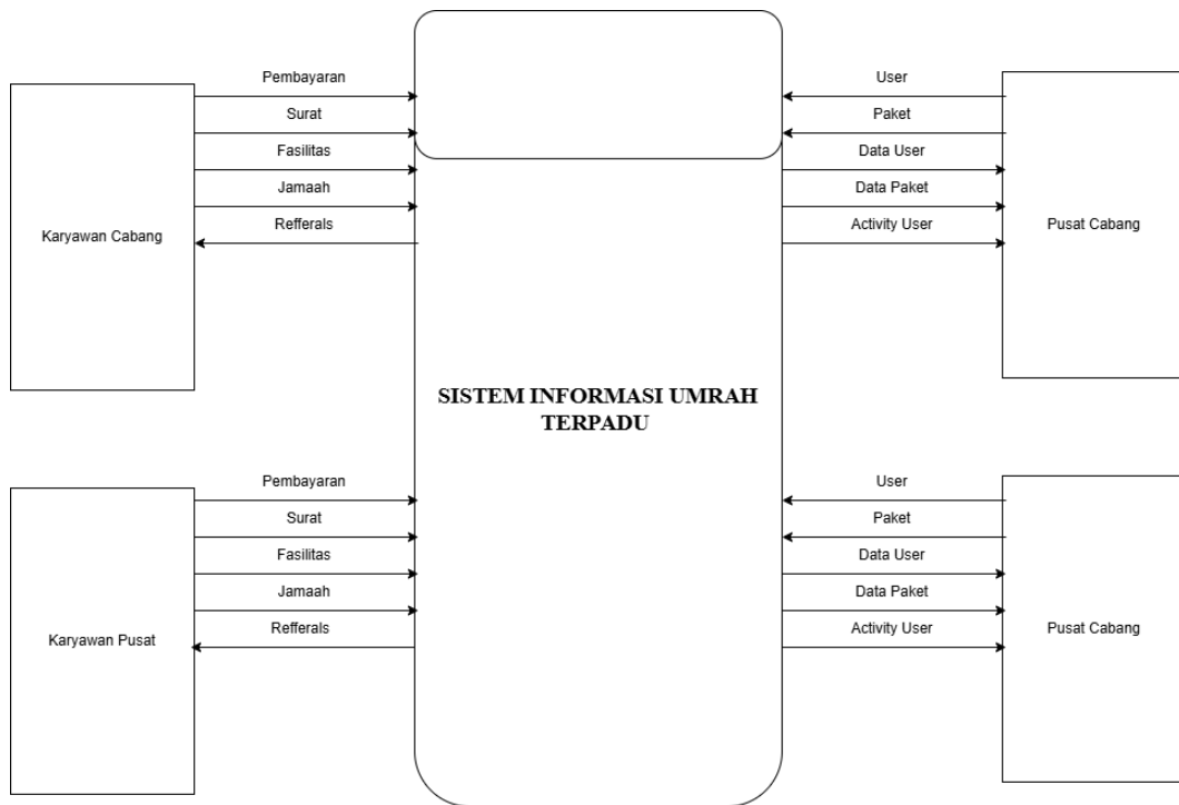
Gambar 4.28 Diagram Konteks
